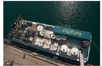
CapturaのDirect Ocean Capture装置
